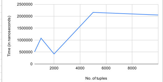
Join - LinHashMap (d)
