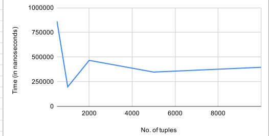
Select - LinHashMap (d)
